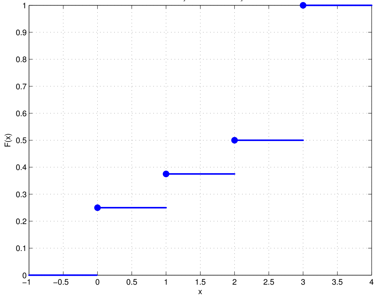
Função Distribuição
